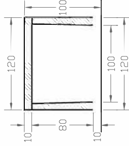
SEZIONE B-B
