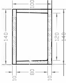
SEZIONE A-A
