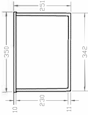
SEZIONE A-A
