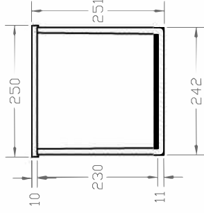
SEZIONE B-B
