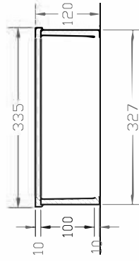
SEZIONE A-A
