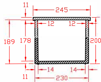
SEZIONE A-A
