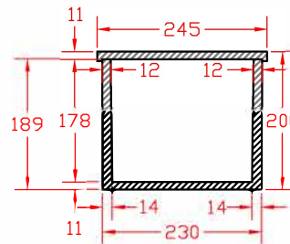
SEZIONE B-B
