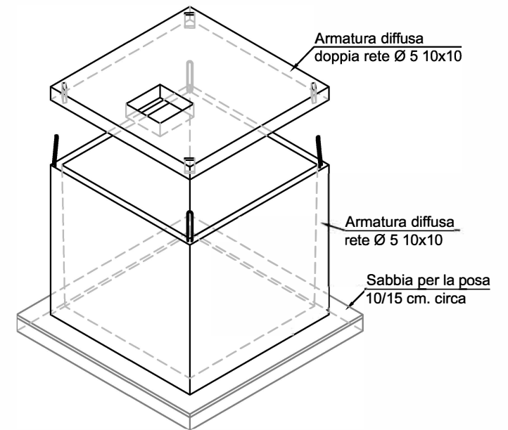
VISTA ASSONOMETRICA
